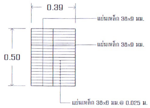
ขยายฝาปิดรางระบายน้ำ มาตรฐาน No Scale
