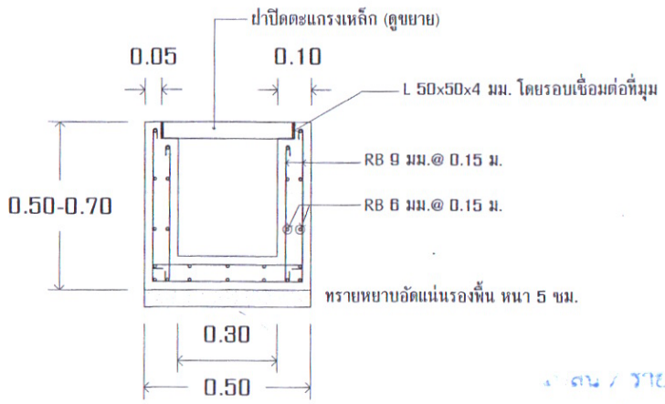
ขยายวางระบายน้ำ คสล. มาตรฐาน No Scale
