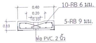
ขยายฝารางระบายน้ำ มาตราส่วน No Scale
