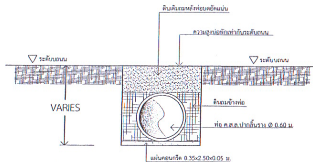
รูปตัด B มาตราส่วน No Scale
