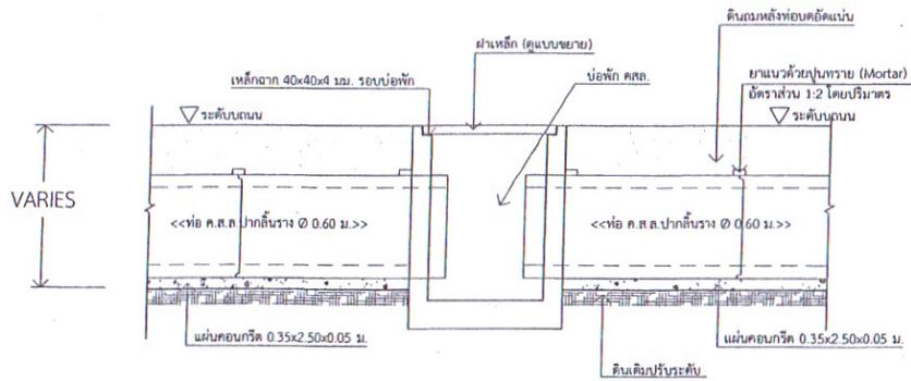
รูปตัด A มาตราส่วน No Scale
