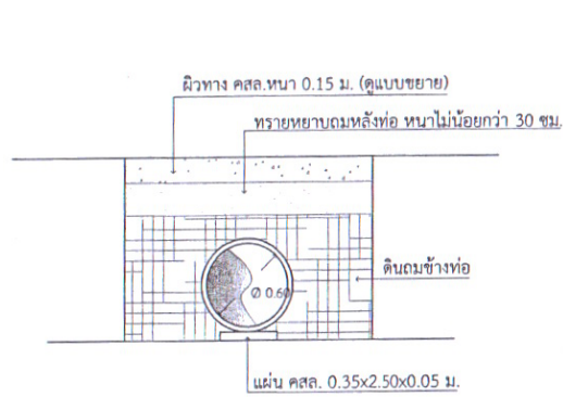
ขยายจุดตัดท่อลอดถนน มาตราส่วน No Scale
