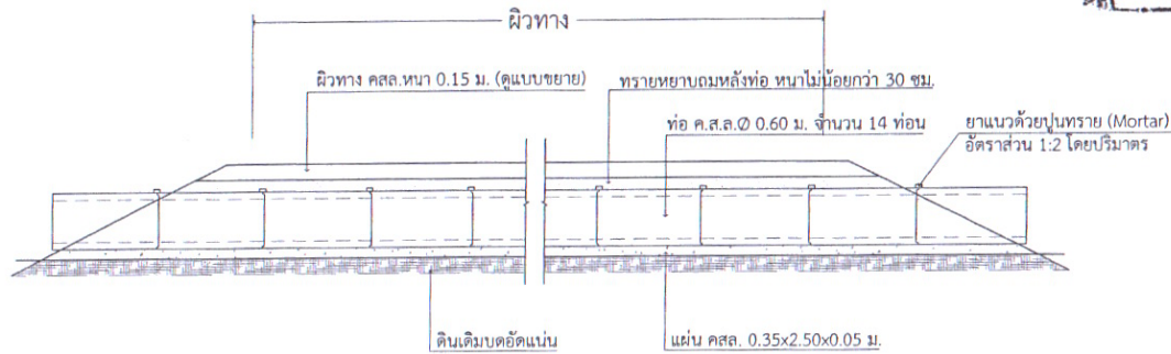
รูปตัดการวางท่อ ค.ส.ล. 0.60 ม. มาตราส่วน No Scale
