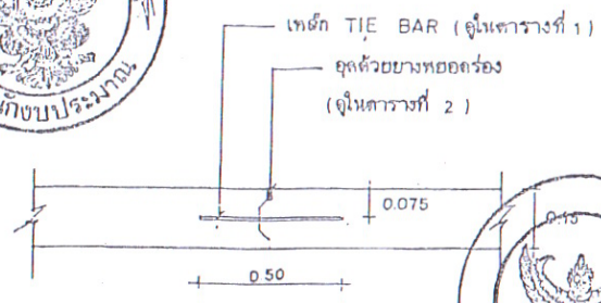
LONGITUDINAL JOINT
